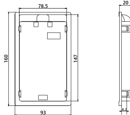
安装座
